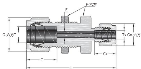
英制縮徑雙卡套穿板直通
