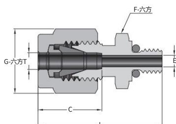
英制雙卡套陽螺紋直通
