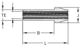
雙卡套孔口接頭
