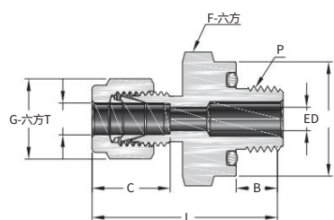
英制雙卡套陽螺紋直通
