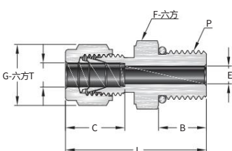
轉接至iso 6149-1 直螺紋凸台
