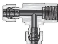
雙卡套主管陰螺紋三通
