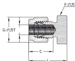
英制管帽
