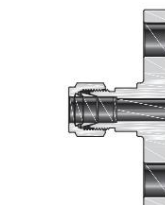
雙卡套法蘭接頭
