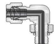
雙卡套可定位陽螺紋彎頭
