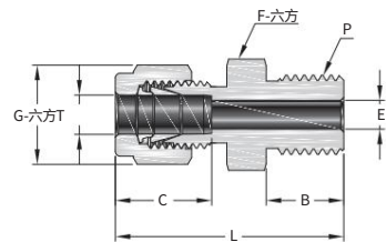
英制雙卡套陽螺紋直通
