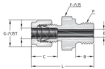
雙卡套陽螺紋直通
